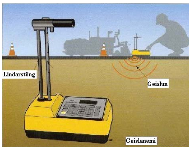
Mynd 1: Troxler tæki. Geislaálaginn mælir gammageislun og nifteindageislun sem endurvarpast úr jarðvegi.
